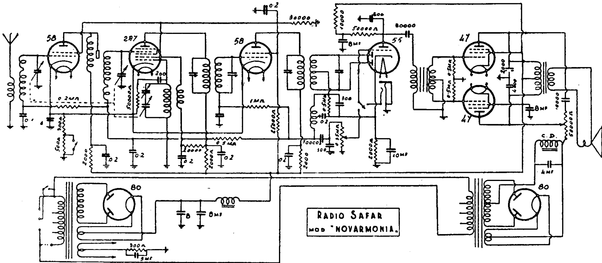
RADIO SAFAR. — Modello « Novarmonia ». • Produzione 1934.
